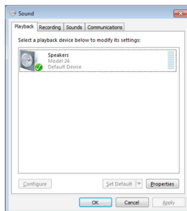
Pantalla Windows 7
