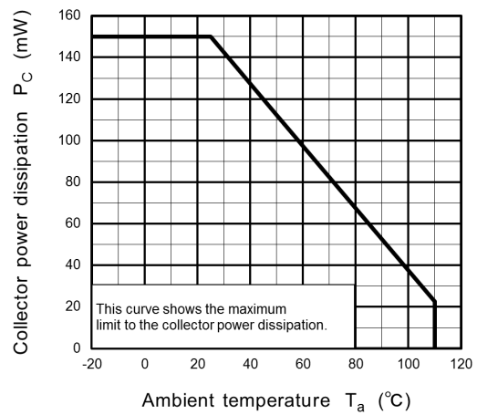
Fig. 11.2 P_C - T_a
