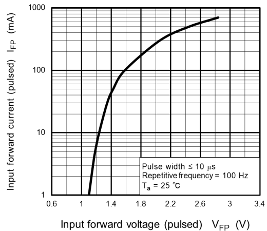
Fig. 11.6 I_{FP} - V_{FFP}
