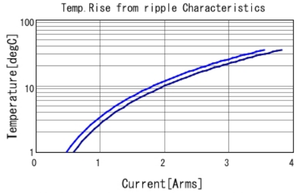
GRM188R61E225KA12 Temp. rise — 500kHz — 1MHz
