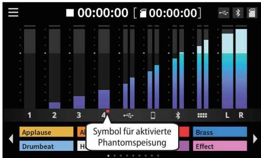
Kanal 3 ist auf ein Kondensatormikrofon eingestellt (Phantomspaltung eingeschaltet)
