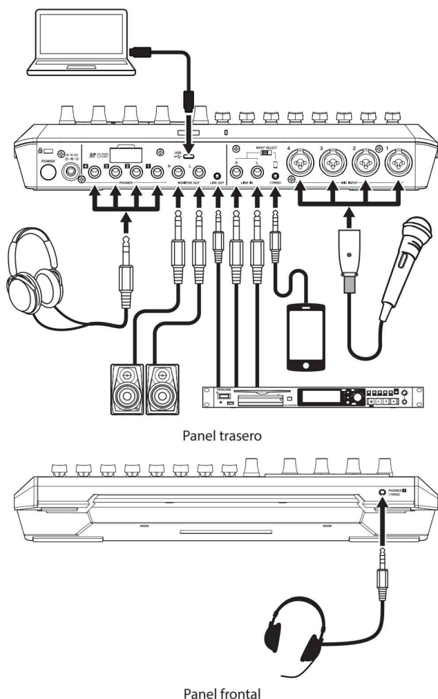
Ejemplo de conexión
