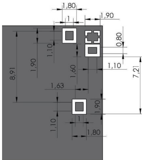
Top Layer
