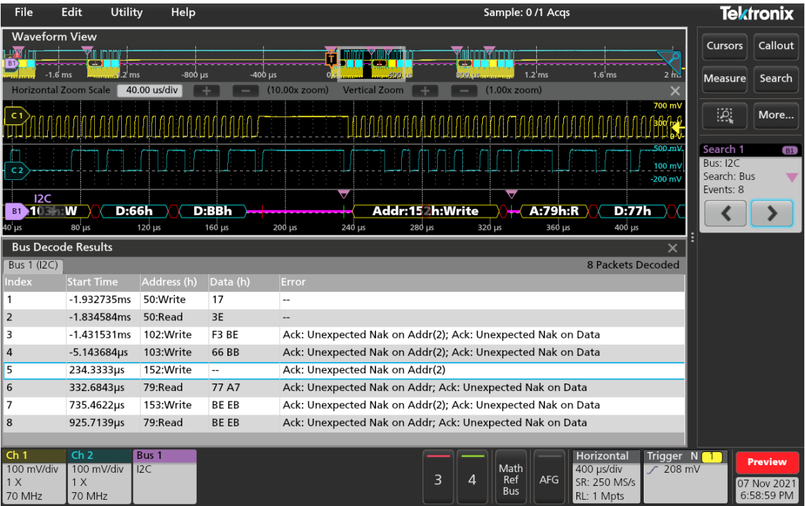
Una forma de onda de bus proporciona paquetes descodificados correlacionados con el tiempo mientras que la tabla de descodificación de bus presenta los distintos paquetes de toda la adquisición, la búsqueda se puede utilizar para navegar
