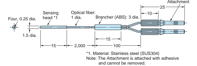
E32-D25XB
