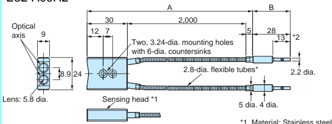
E32-A09H2
