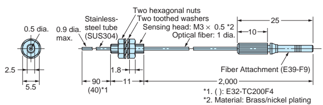
E32-T24 E32-T24R
