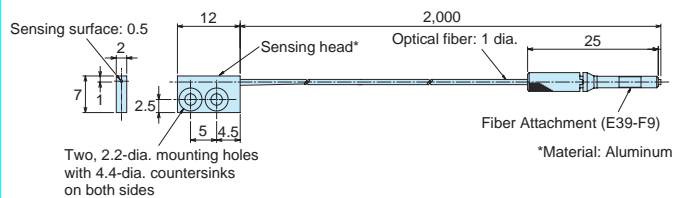
E32-TC200(F4) E32-TC200F(F4R)
