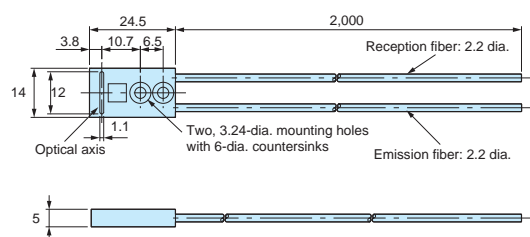
E32-A09 E32-A09H
