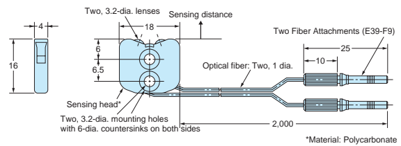
E32-L25A
