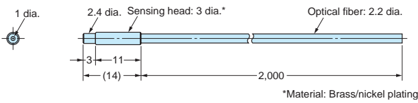
E32-T12 E32-T12R
