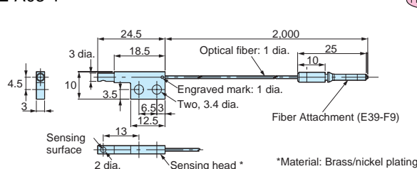
E32-A03-1
