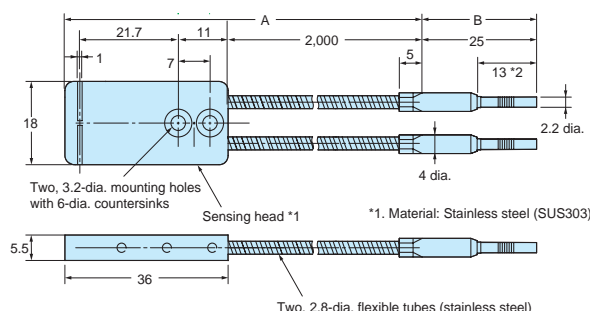
E32-L66
