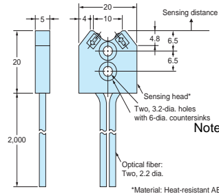
E32-L25A
