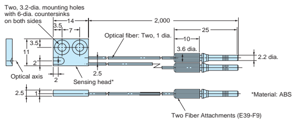
E32-L24L
