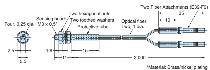
E32-D22B
