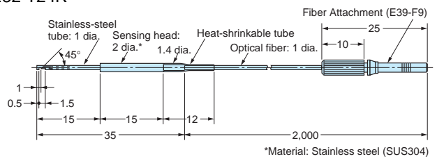
E32-T24 E32-T24R
