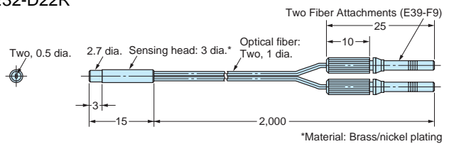
E32-D22 E32-D22R
