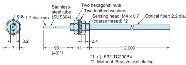
E32-T14L E32-T14LR
