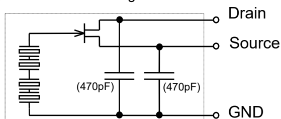
図3. 内部回路構成
