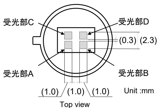
図 2. 受光部寸法
