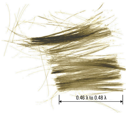
Fig. 17: Chaff
