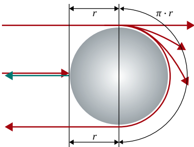
Fig. 37: Creeping wave
