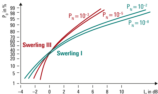
Fig. 35: Swerling targets
