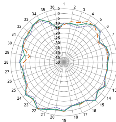
XZ-Plane Gain
