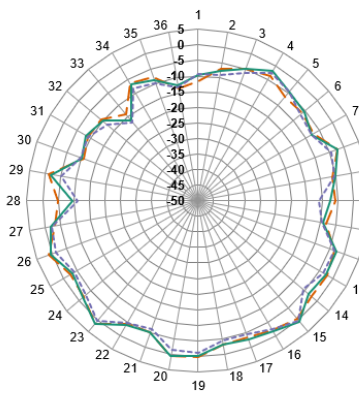
YZ-Plane Gain
