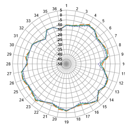
YZ-Plane Gain
