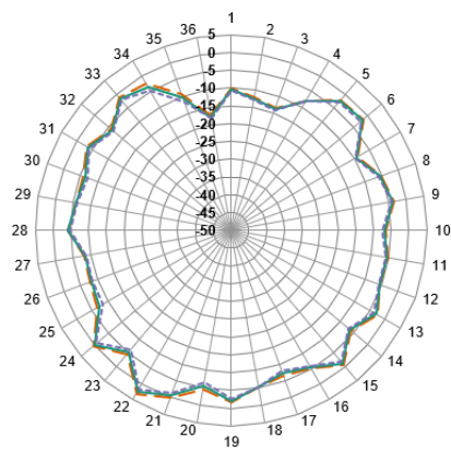
XZ-Plane Gain
