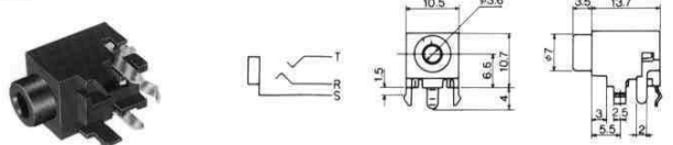
No.MX-362GL (φ3.5) STEREO
