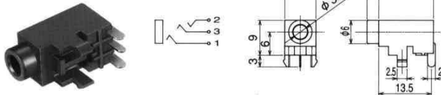
No.MX-345GLB ( \phi 3.5 ) STEREO Net Weight : 1 gr.
