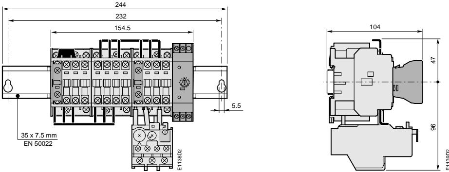
YKA 9-30 ... YKA 16-30 + TA 25
