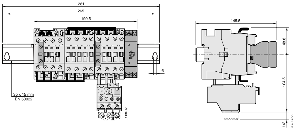
YKA 30-30 + TA 25
