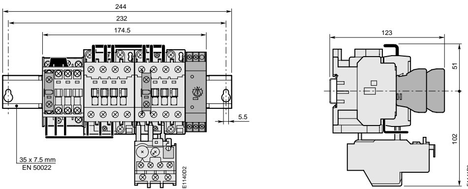
YKA 26-30 + TA 25
