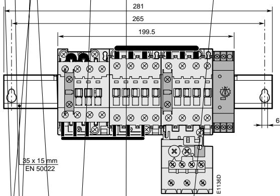
YKA 40-30 + TA 42
