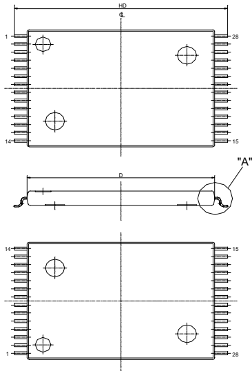
TSOP - 28
