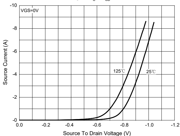
Fig. 5 - I_S - V_{SD}
