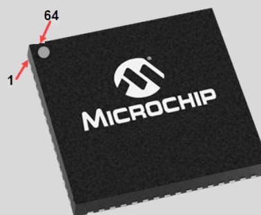
Figure 4-6. VQFN
