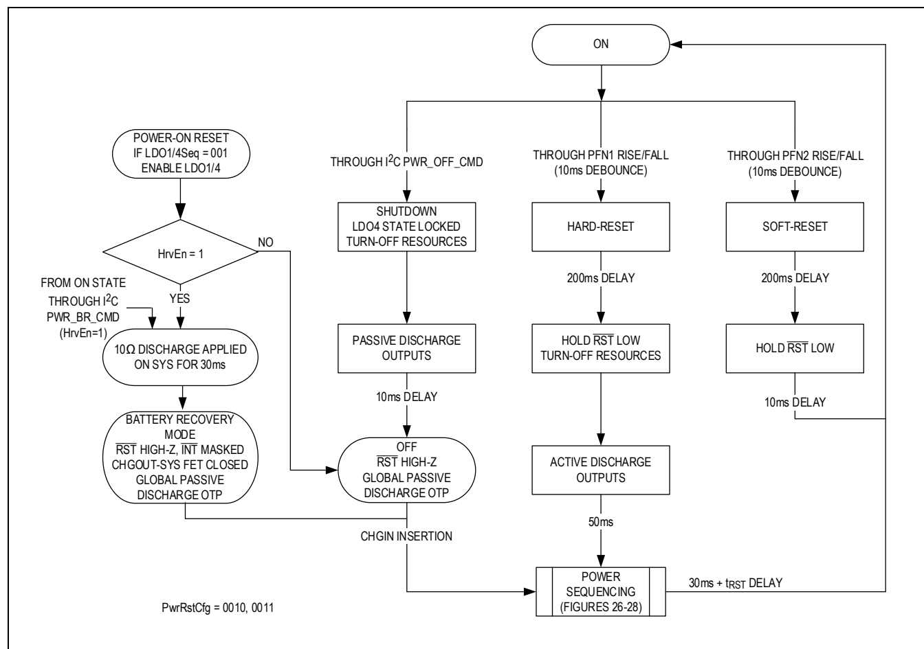
Figure 14. PwrRstCfg 0010, 0011
