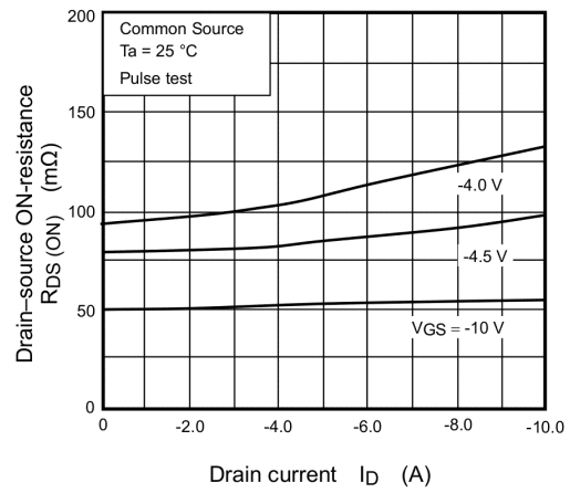
Fig. 8.4 R_{DS(ON)} - I_D
