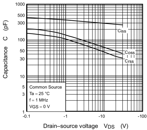
Fig. 8.7 C - V_{DS}
