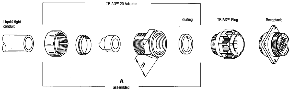
TRIAD 20 Conduit adaptor
