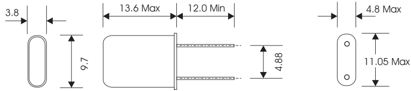
HC-49/U
